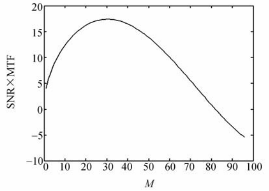
图 3 不同积分级数 M 下 SNR \times MTF 值 ( \phi' = 0.007 ( ^\circ )/s)
