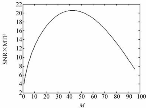
图1 不同积分级数 M 下的 \text{SNR} \times \text{MTF} 值( \phi' = 0.005 \text{ (}^\circ\text{)/s} )
